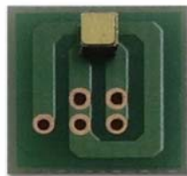
評価用センサーボード CMN200-K
